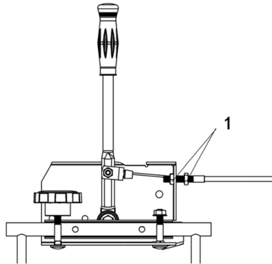
Adjust cable
