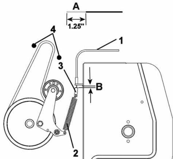
Adjust cable
